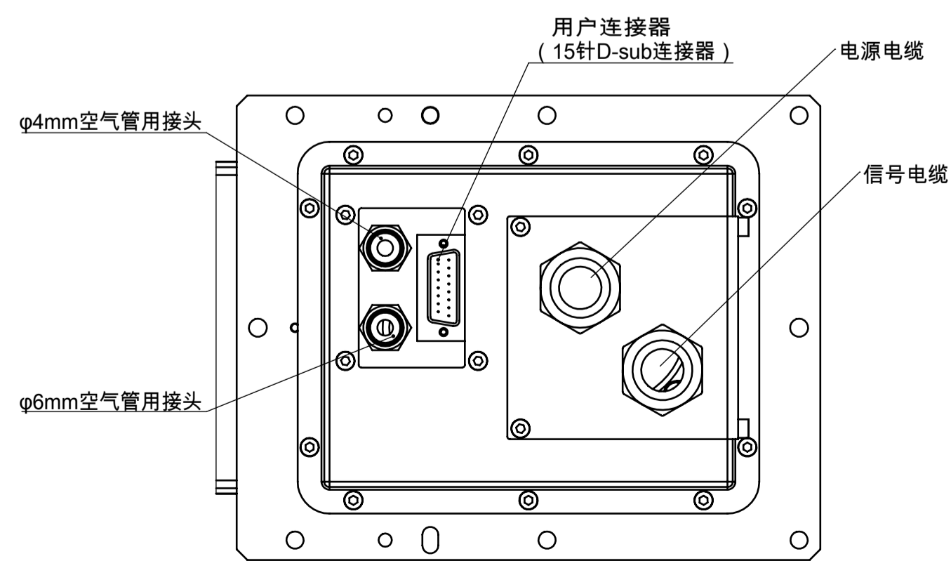
C部视图
