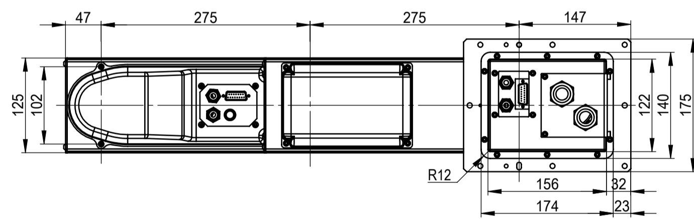
B部视图
