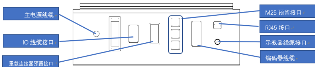
图 1.5 对外接口
