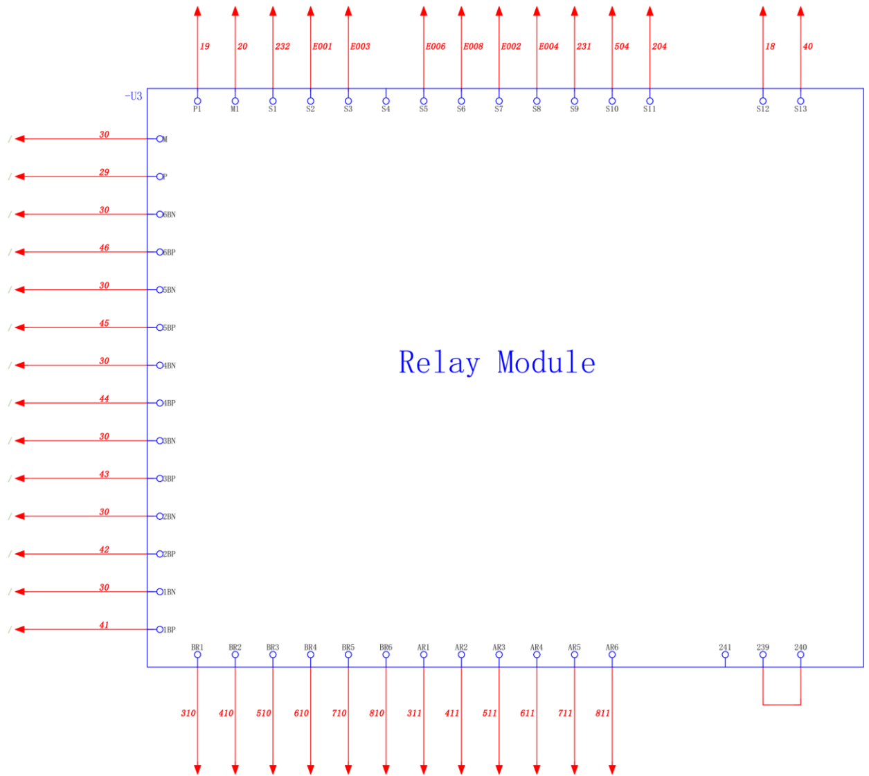
图 3.23 继电器模组
