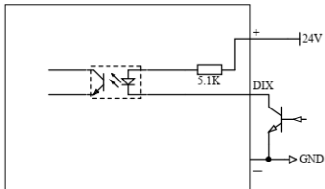
图 3.15 DI NPN 型接线图
