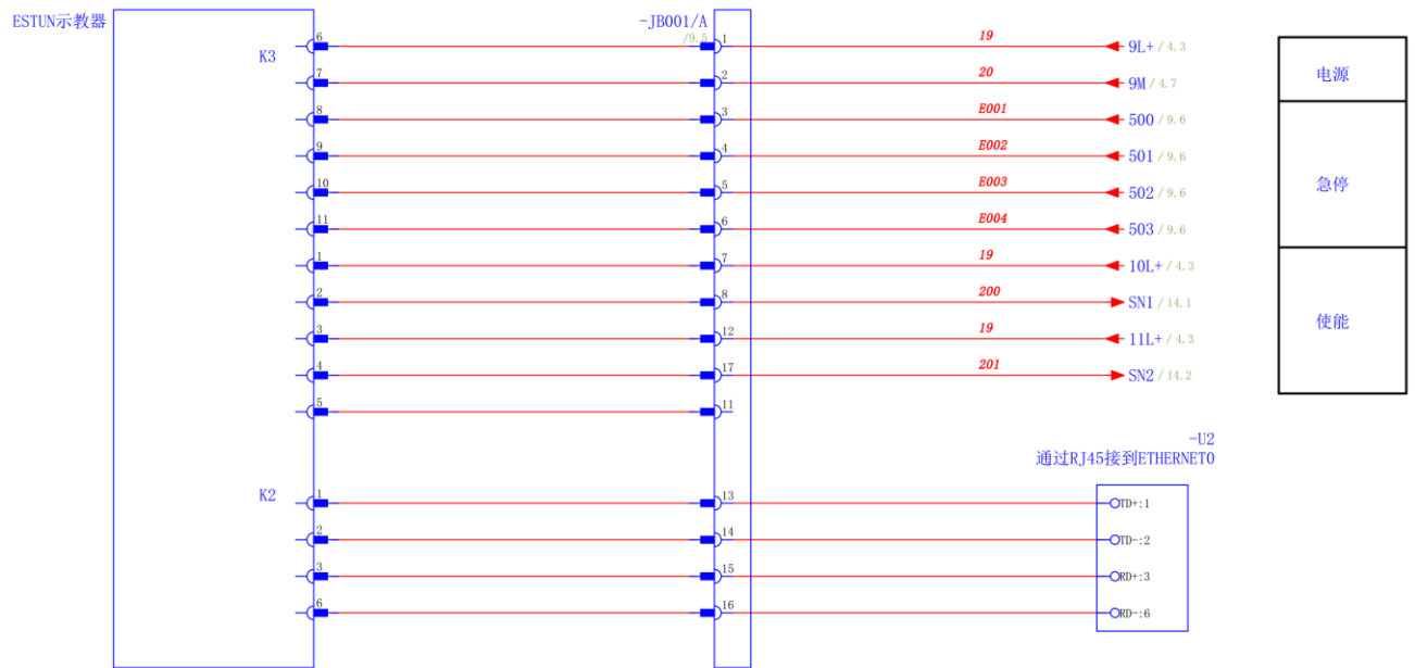
图 3.11 示教器接线
