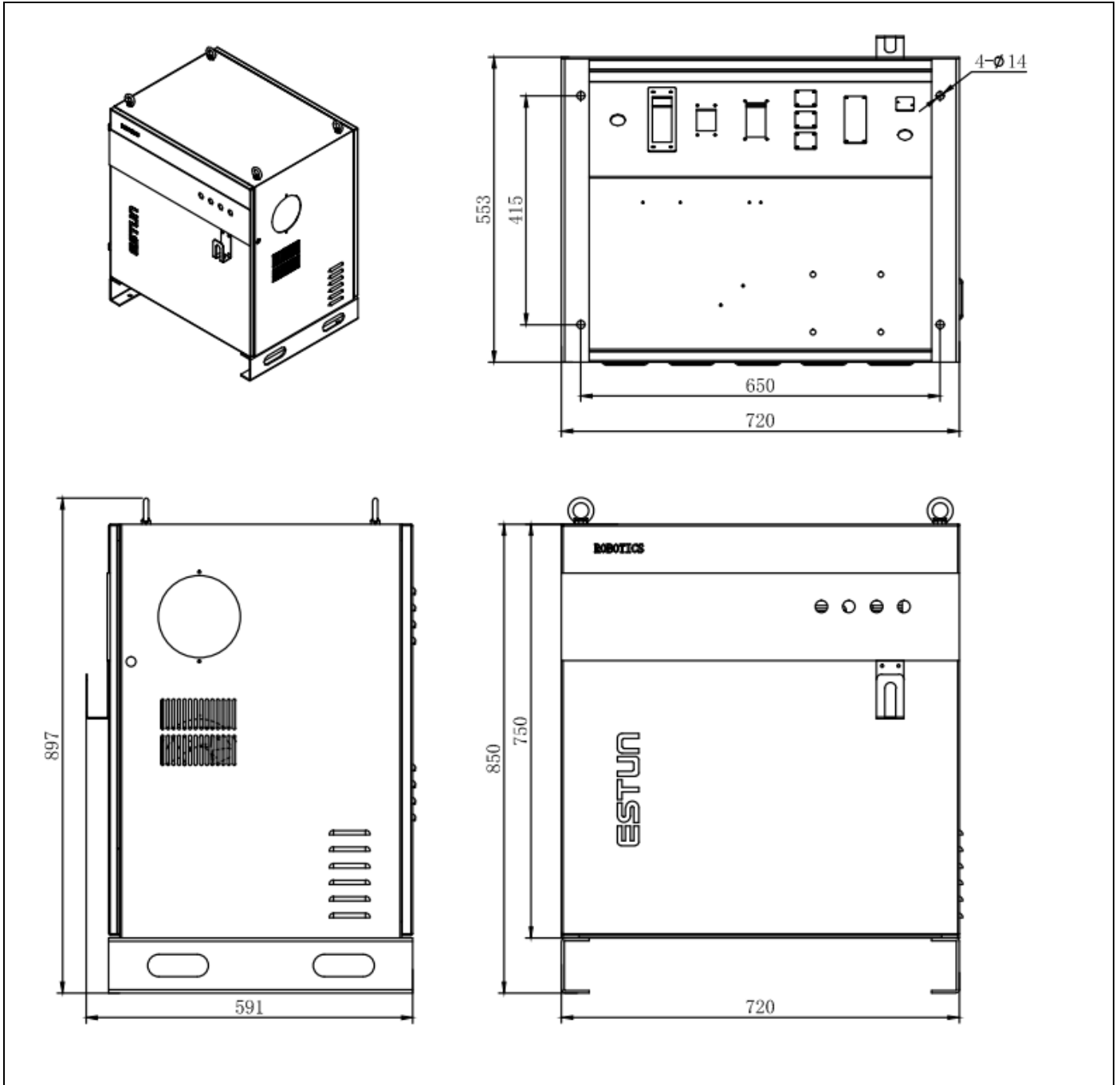
图 1.6 产品尺寸图
