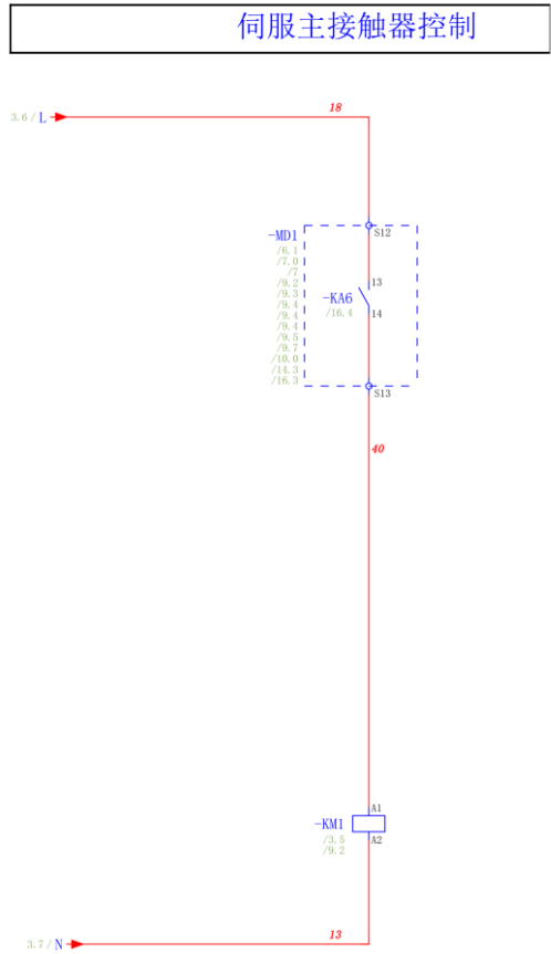
图 3.9 AC 220V 控制回路
