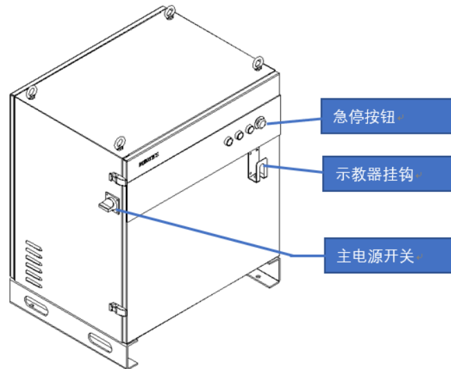
图 1.3 外观说明
