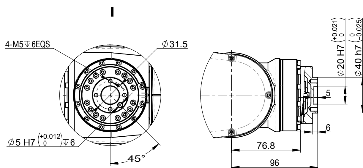
底座安装接口
