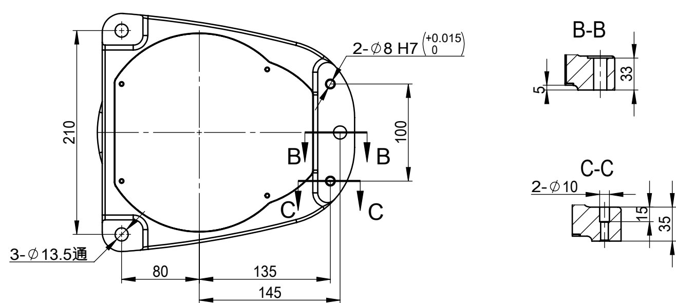
底座安装接口
